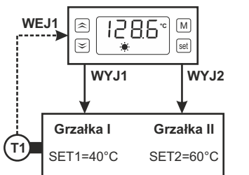
Piec z dwoma stopniami grzałek
