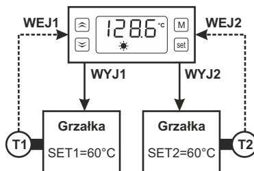
Dwa oddzielne piece
