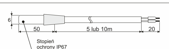
Rys.4. Wymiary czujnika przewodowego.
